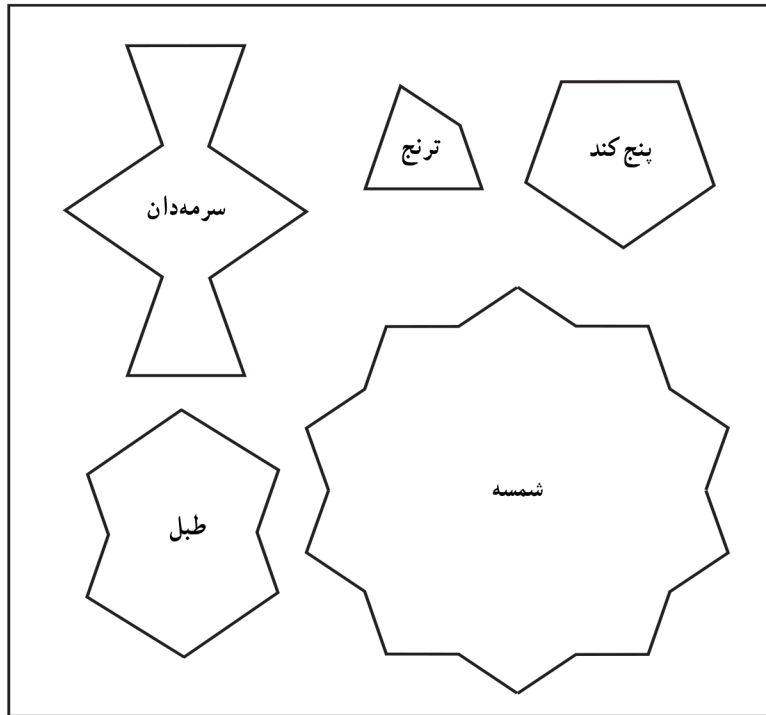
شکل ۳-۷- آلت گره ها، از گره سرمه دان چهار شمشه
